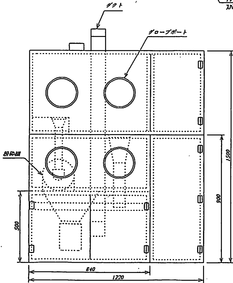
立面図
