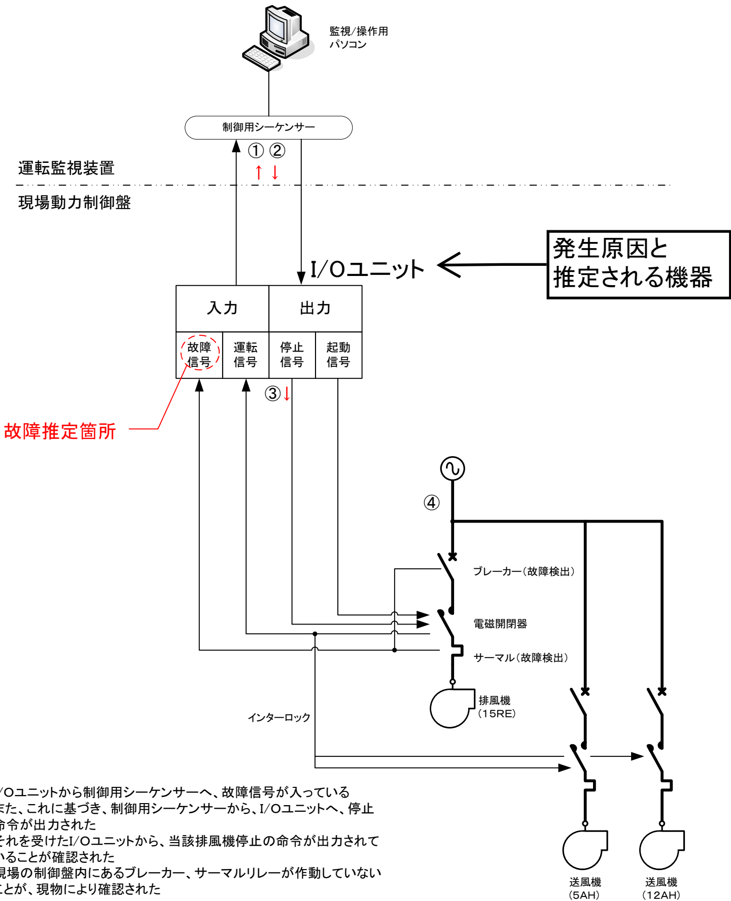
当該排風機に係る監視制御系統図
