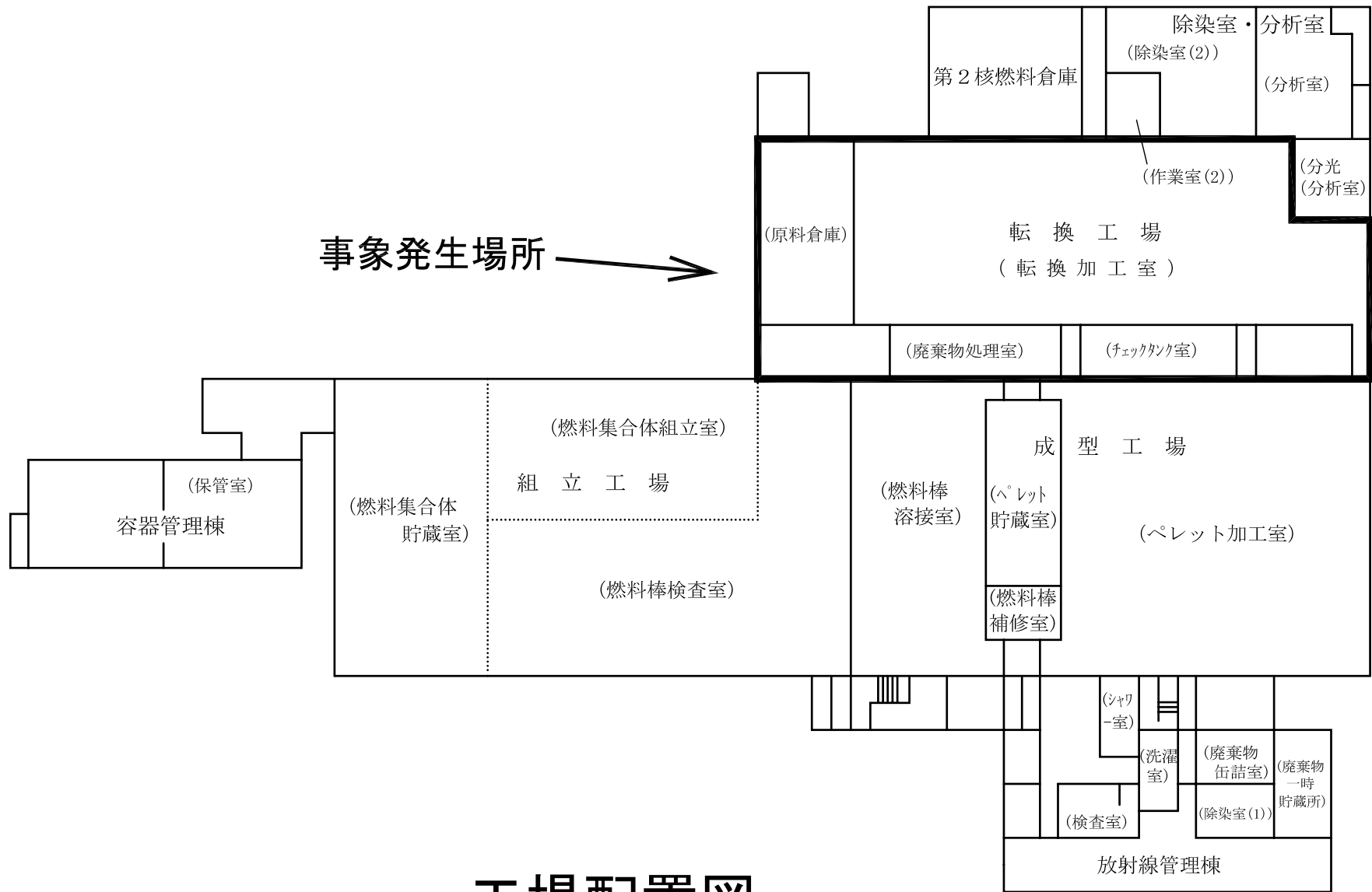
工場配置図
